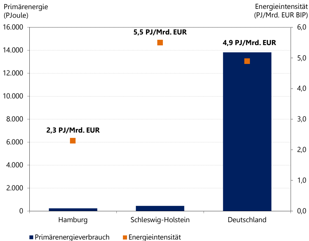
ABBILDUNG 84: ENERGIEINTENSITÄT 2013
